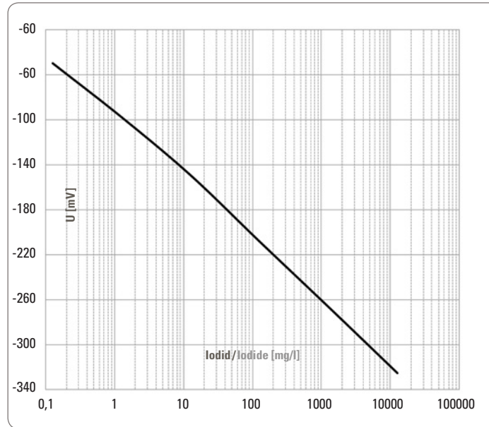
Steilheit/Slope
